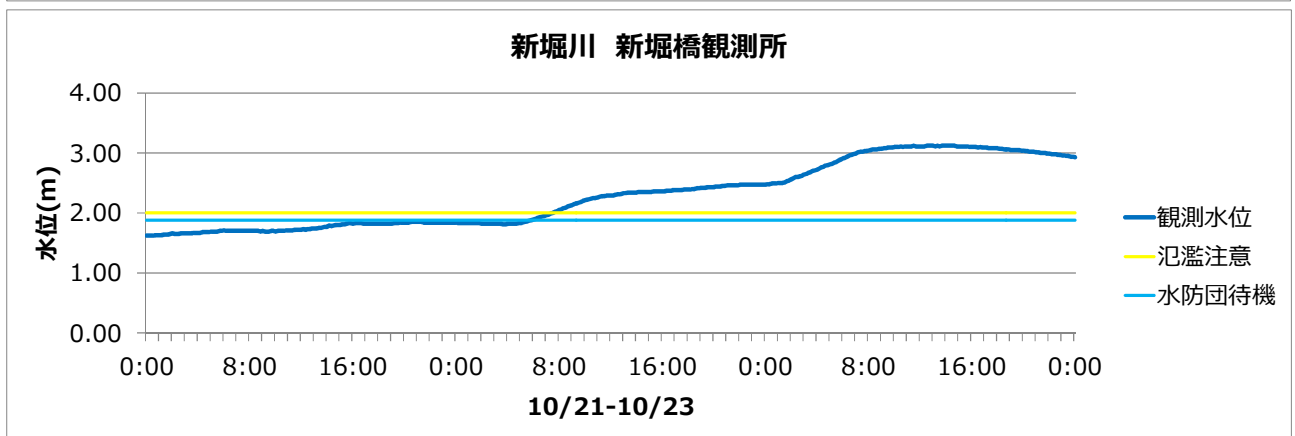
図7 時系列の水位状況(各水位観測所)
