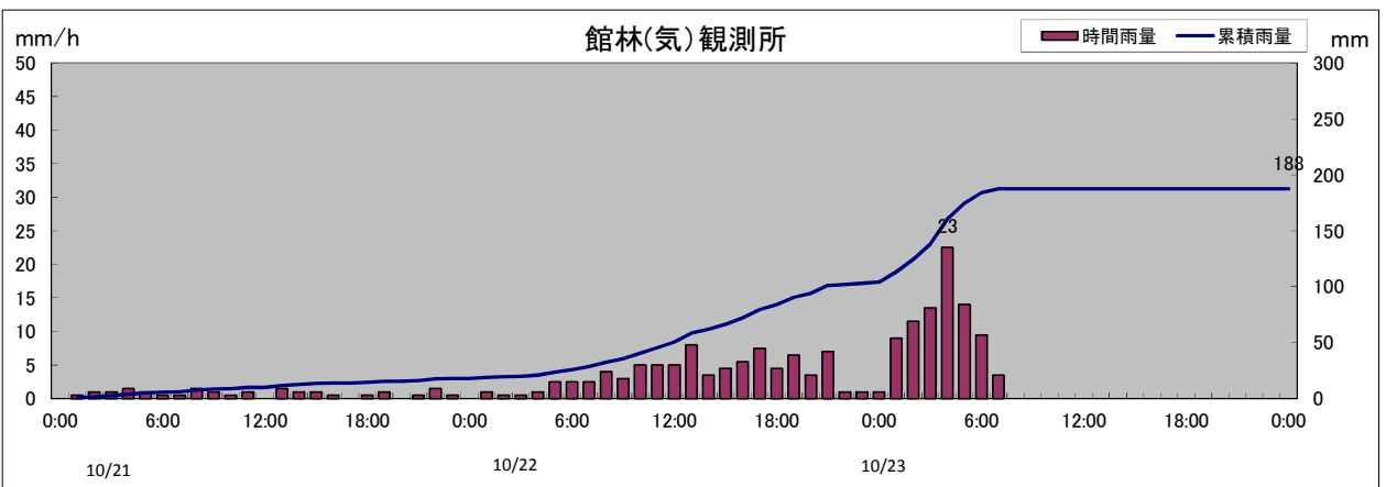
図6 時系列の降雨状況(菱町・太田・伊勢崎・館林の各雨量観測所)
