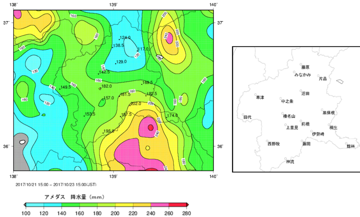
図4 アメダス期間降水量(単位:mm 10月21日15時~23日15時)
