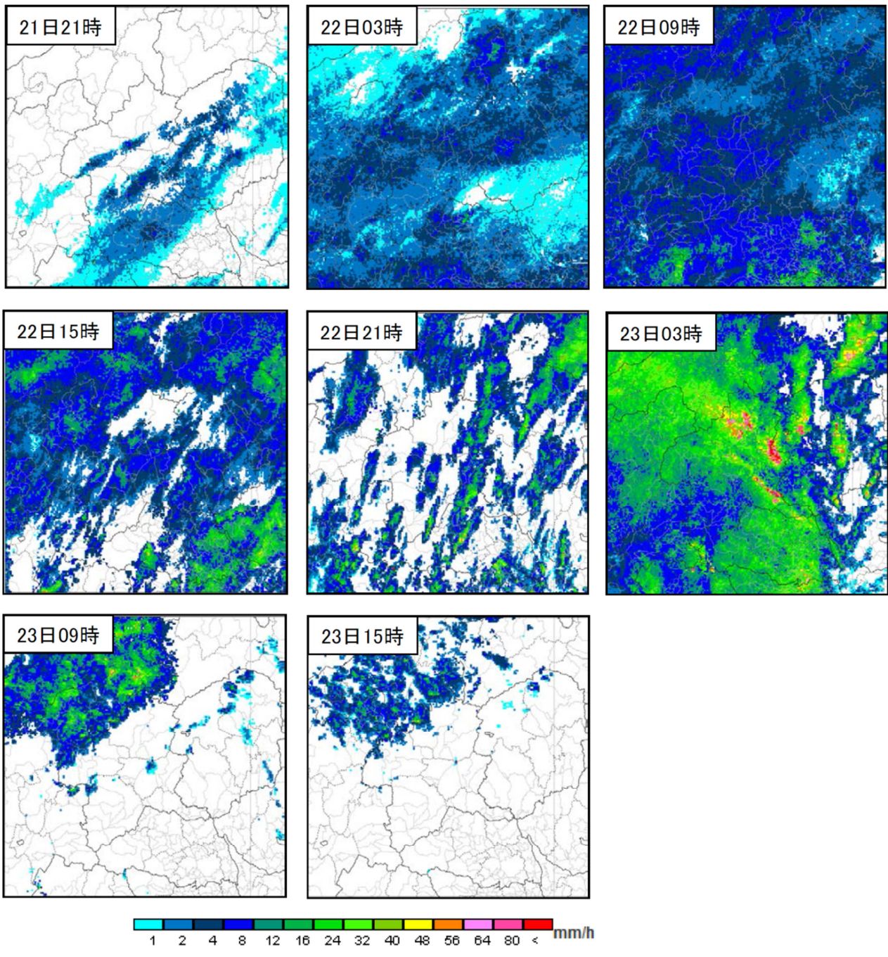
図3 レーダー画像 (10月21日21時から10月23日15時まで:間隔6時間)
