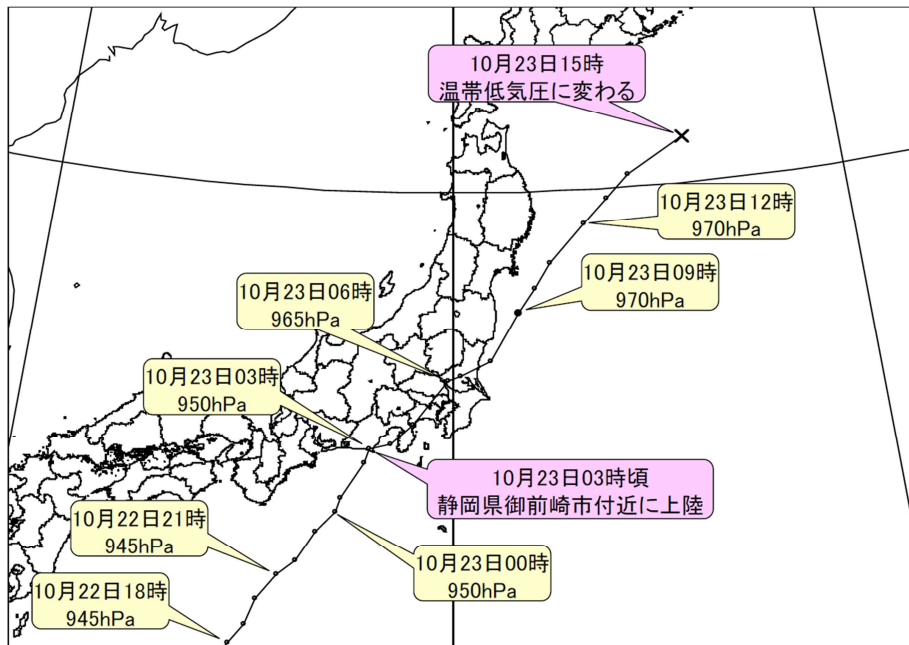
図1 台風第21号経路図（速報解析）
