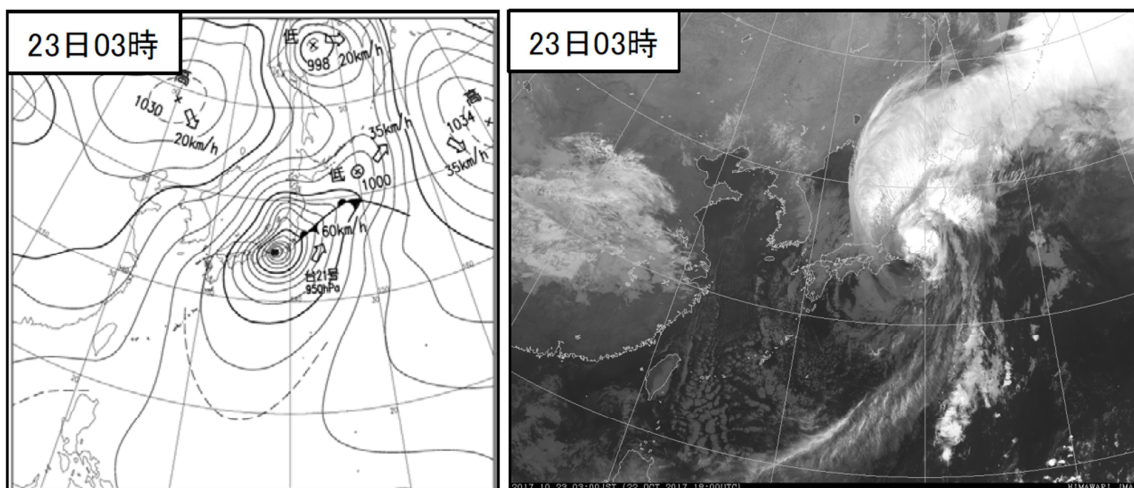
図2 台風第21号天気図・気象衛星写真(10月23日3:00)
